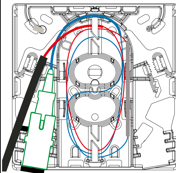
Fixation du câble à gauche Left fixation cable
